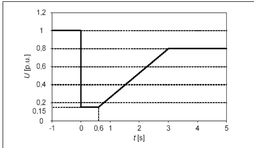
Rys. 1. Charakterystyka wymaganego zakresu pracy elektrowni wiatrowej w przypadku wystąpienia zakłóceń w sieci.
